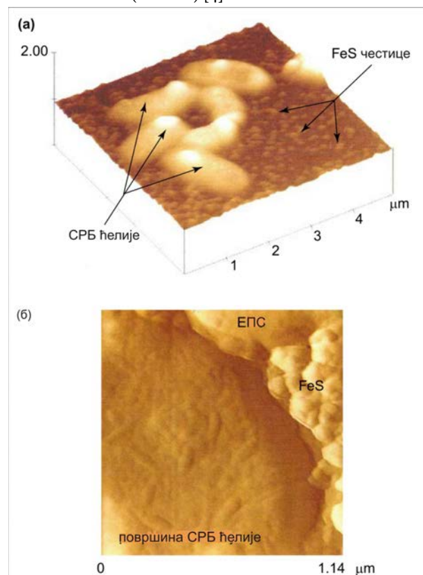
Слика 1. Микроскопија атомских сила биофилма старог 14 дана формираног од стране морских сулфат-редукујућих бактерија СРБ Desulfovibrio alaskensis на површини AISI 316 нарђајућег челика. (а) Гвожђе сулфид (FeS) честице се виде распоређене на површини челика и б) веома су тесно повезане са бактеријама и екстрацелуларним полимерним супстанцама (ЕПС) које излучују ћелије [4].
