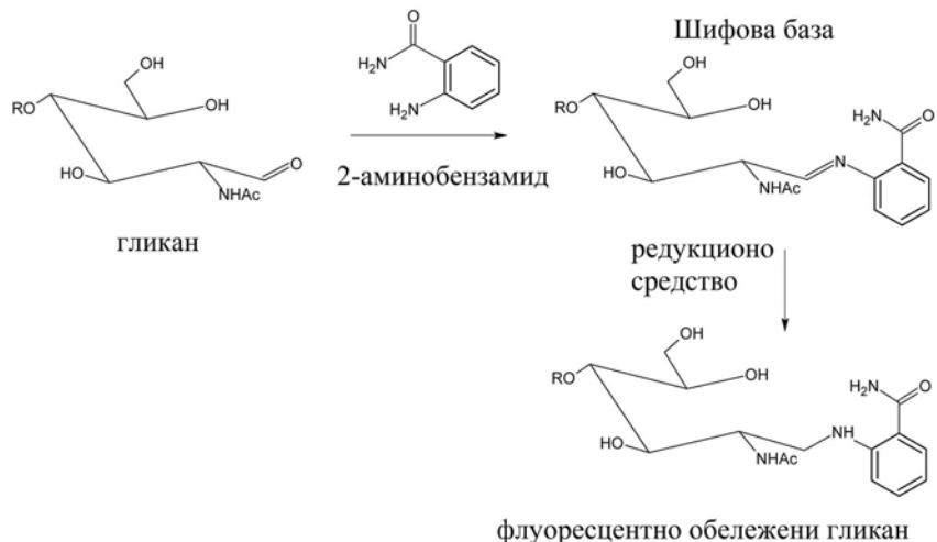
Слика 6. Обележавање гликана флуоресцентном пробом (2-аминобензамид) у реакцији редуктивног аминаовања [13].
