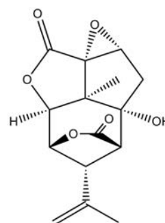
Структура 8. – Пикротоксинин, биљни отров налик стрихнину.
