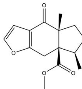
Структура 9. – Пример пингвисана, сесквитерпена из маховина са имуносупресорским дејством.
